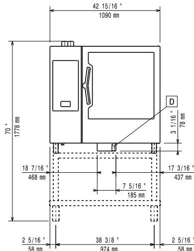
Front aanzicht
